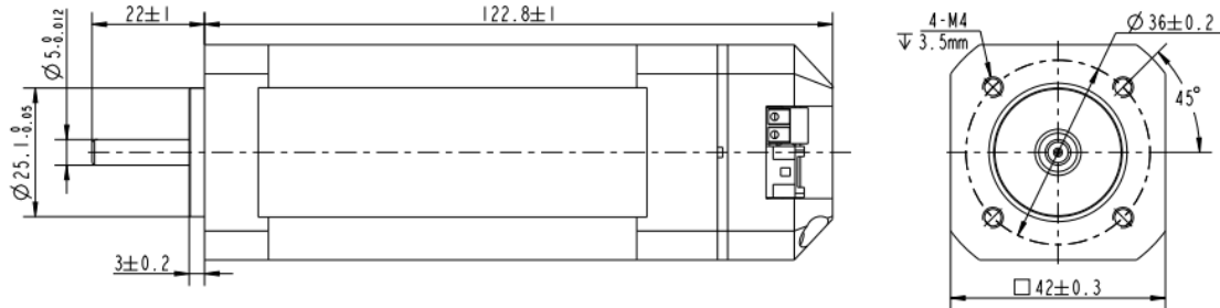
图 1 机械尺寸图
